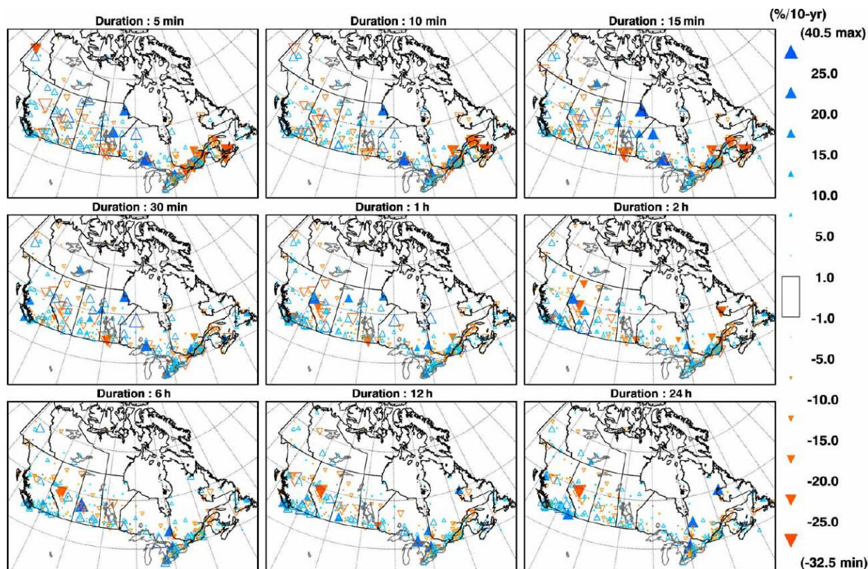
Figure 13. Tendances des pluies extrêmes aux stations météorologiques sur la période 1965-2005, où une station doit posséder au minimum 20 ans de données pour être considérée. Les tendances statistiquement significatives sont indiquées par un triangle plein (Shephard et al. , 2014).
