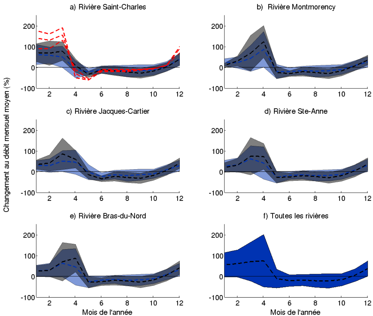
Figure 10. Changements prévus au débit mensuel moyen de quelques rivières de la région de Québec à l'horizon 2050, par rapport à 1971-2000, selon les scénarios climatiques de CMIP3 (bleu) et CMIP5 (gris). La ligne pointillée indique la moyenne. L'analyse suit la méthodologie employée par la Direction de l'expertise hydrique (DEH) du MDDELCC dans le cadre de ses deux éditions de l'Atlas hydroclimatique du Québec méridional (CEHQ, 2013; 2015). À l'intérieur d'une même simulation, la dispersion des résultats inclut la moitié des scénarios climatiques analysés. Les lignes rouges illustrent les résultats de Cochand (2014) à l'horizon 2080.
