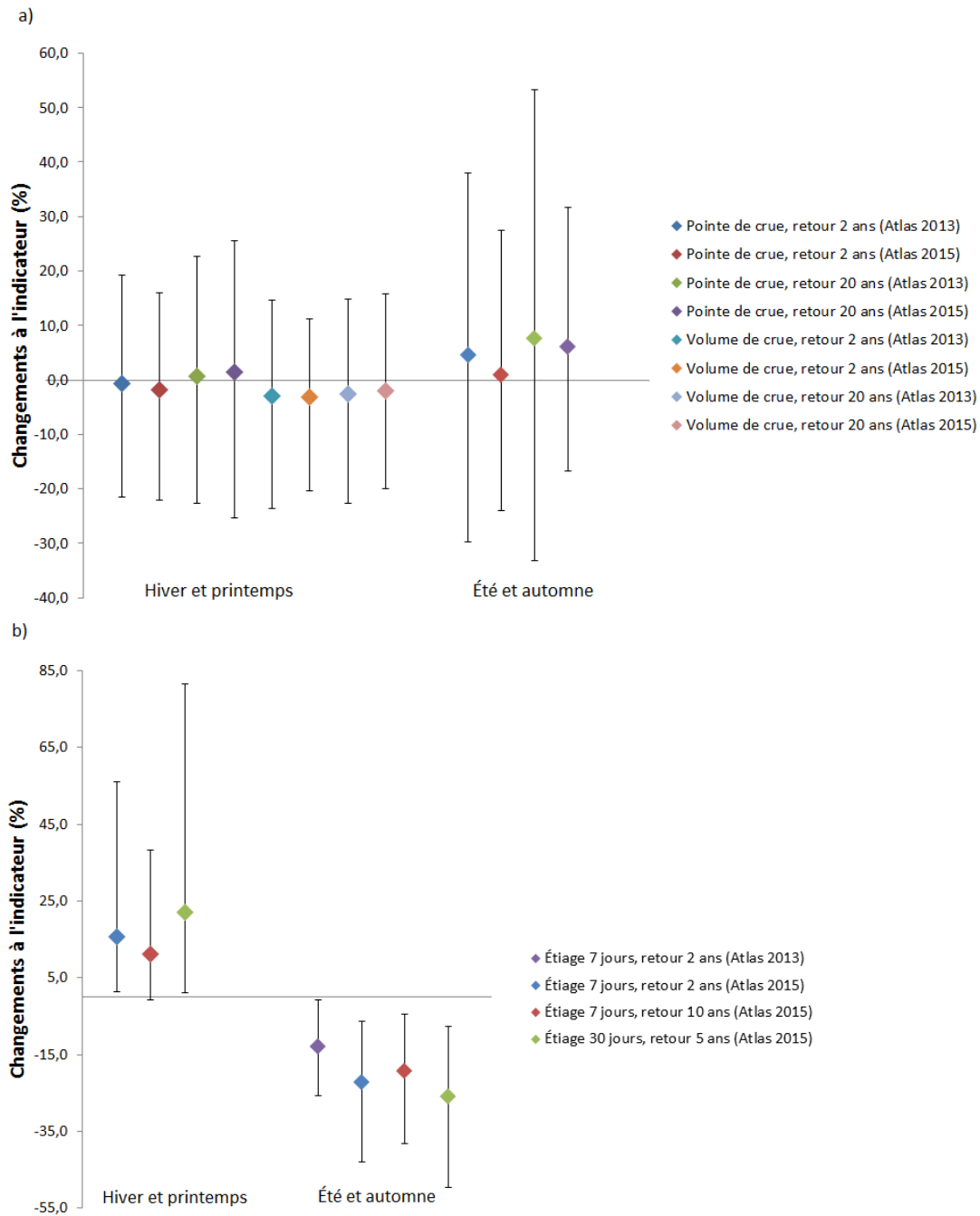
Figure 11. Changements prévus aux débits extrêmes par l'Atlas hydroclimatique du Québec méridional à l'horizon 2050. Les résultats affichés regroupent les rivières Saint-Charles, Montmorency, Jacques-Cartier, Ste-Anne et Bras-du-Nord pour (a) les débits et volumes de crues de périodes 2 et 20 ans et (b) les étiages 7 jours de 2 et 10 ans et étiage 30 jours de 5 ans. Noter que certains indicateurs n'étaient pas analysés dans le cadre de l'édition 2013 de l'Atlas hydroclimatique. Le point indique la moyenne de toutes les rivières et les barres verticales représentent la dispersion des résultats.
