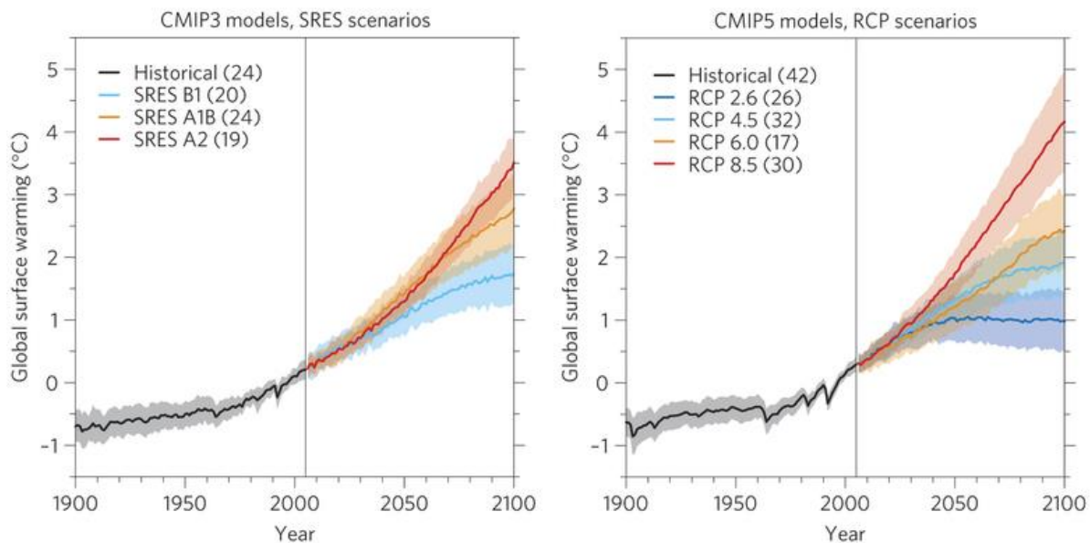
Figure 9. Projections climatiques pour la période 2000-2100. Chaque couleur constitue un scénario d'émissions de GES différents. Les lignes pleines indiquent les moyennes multi-modèles, tandis que la zone ombrée représente un écart-type de déviation relatif à la variabilité interne de chaque modèle. Le nombre entre parenthèses indique le nombre de simulations utilisées. (Knutti et Sedláček, 2013).
