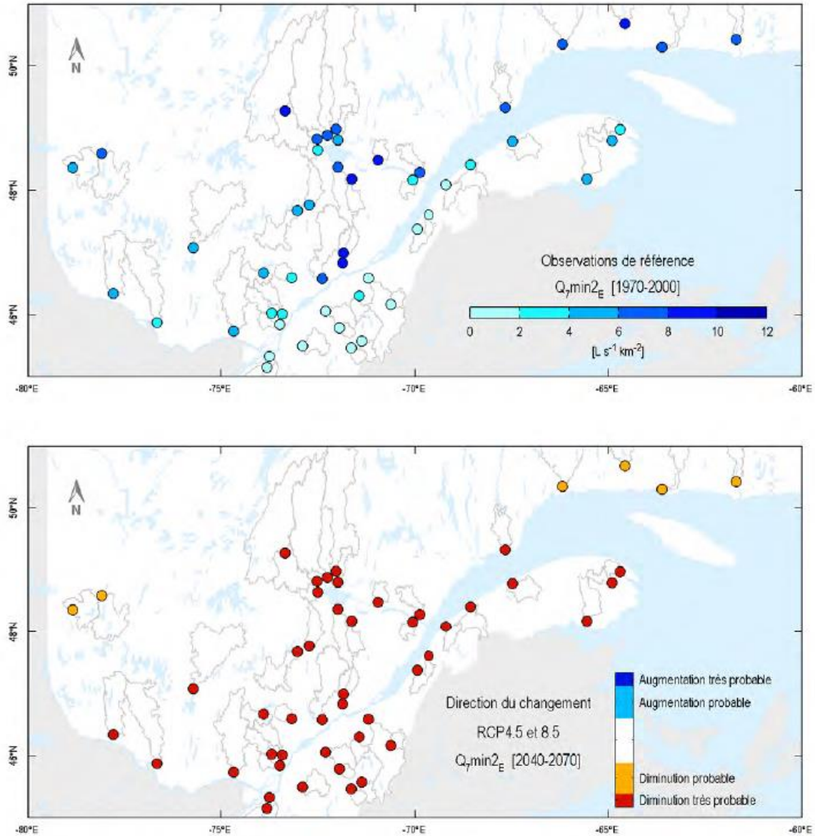
Figure C.3. Étiages estivaux, débit moyen sur 7 jours, récurrence 2 ans (CEHQ, 2015).
